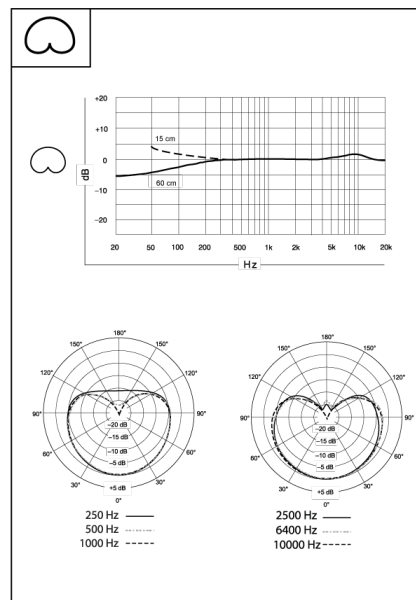
Nierencharakteristik
